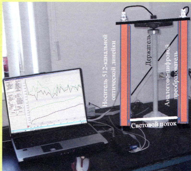
Общий вид 512-канальной МФАИМС
