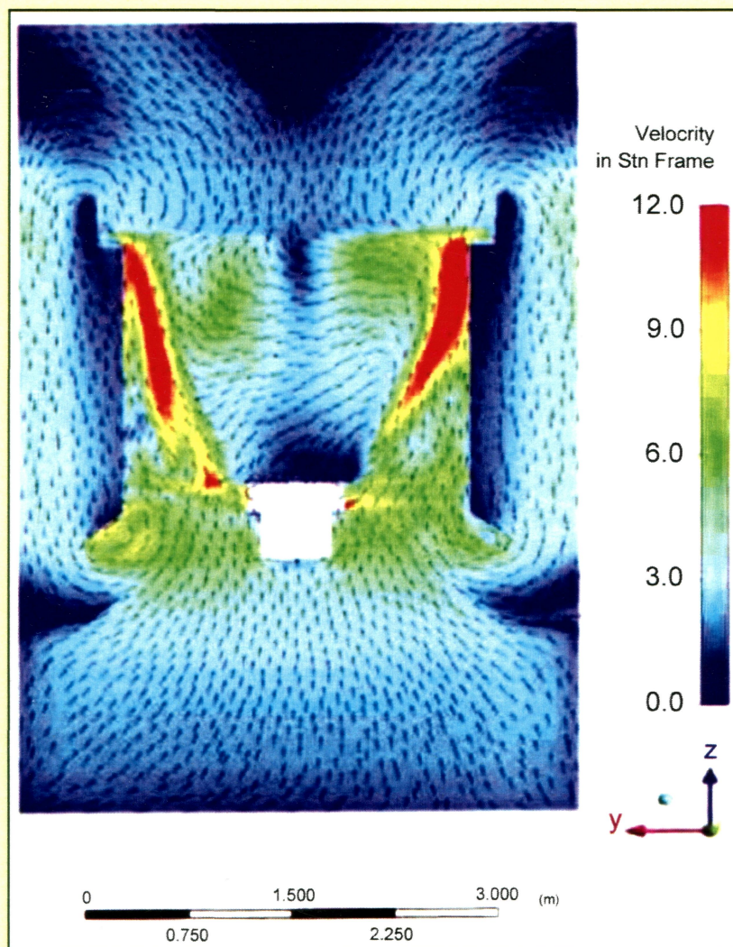
Рис. 1. Структура течения газа в плоскости диффузоров АВО
