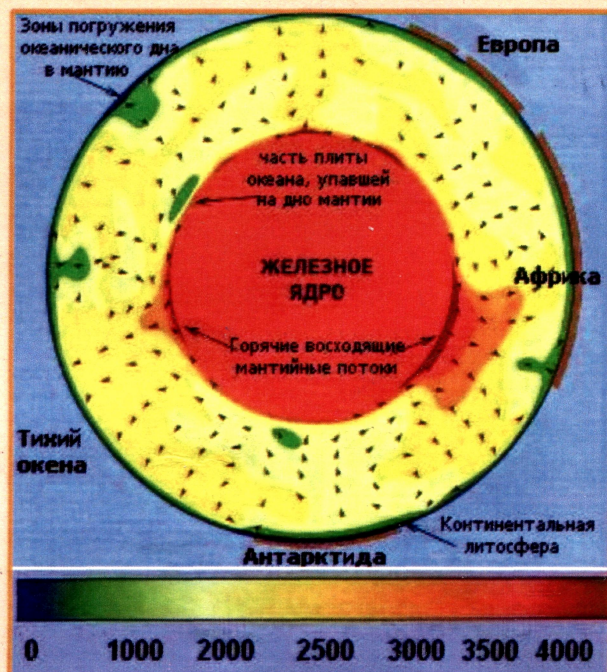
Рис. 2. Современное представление теплового портрета Земли
