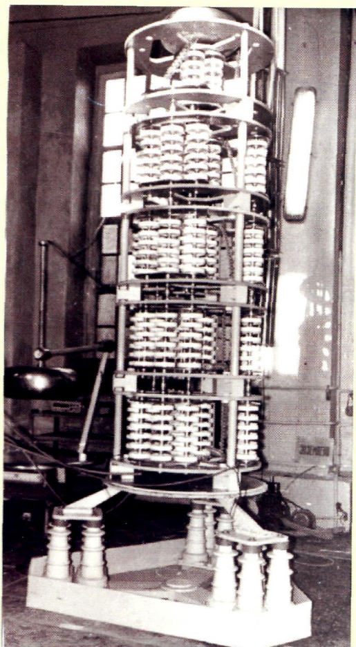
ППВ-750-10 (750 кВ, 10 МА)
