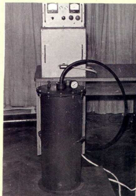
ПВС-160-0,6 СТ (160кВ, 0,6МА)
