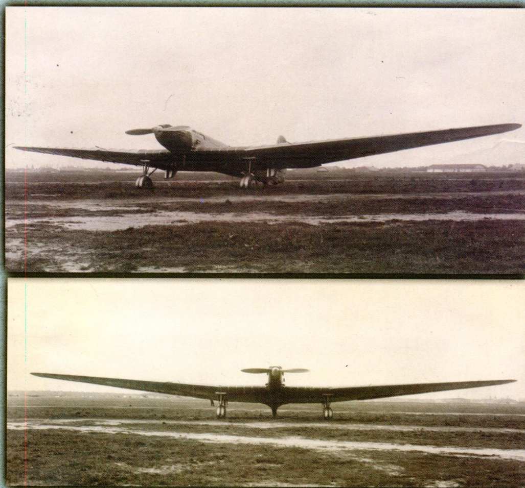
Самолет РД-2 после полета. ЦАГИ. 19 сентября 1934 г. Филиал РГАНТД. Ф.Р-217.Оп.3-1. Д.29. Л.1
