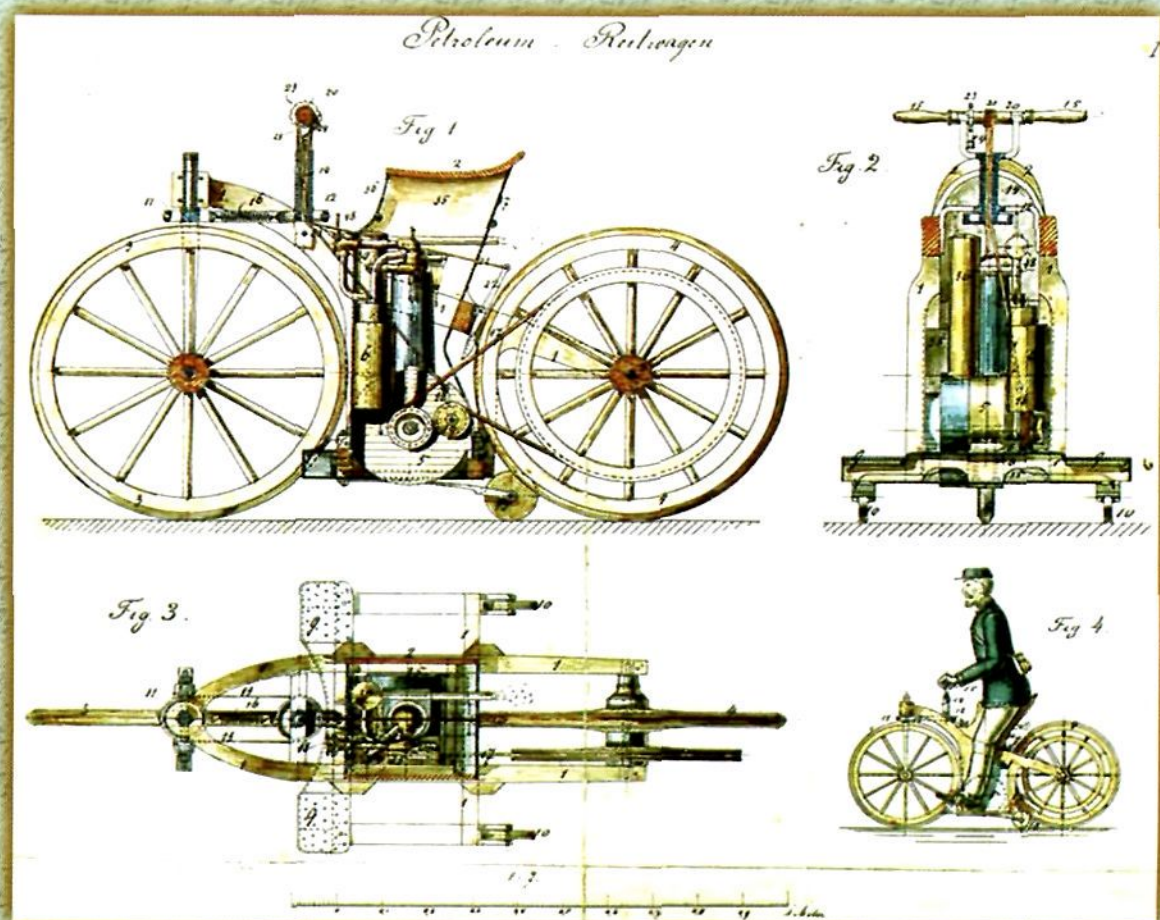
Рис. 2. Чертежи из немецкого патента Г. Даймлера ДРП 34926 от 3 апреля 1885 г.
