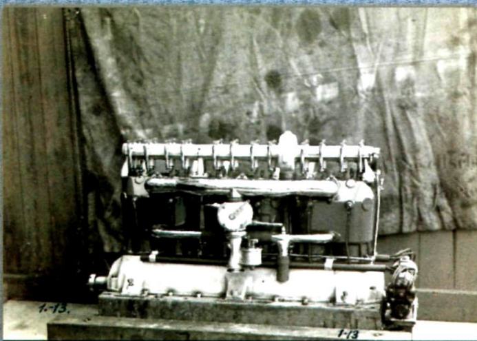
Рис. 2. 150-сильный двигатель конструкции Луцкого. Вид со стороны карбюратора (1914). Фотография из архива РАН
