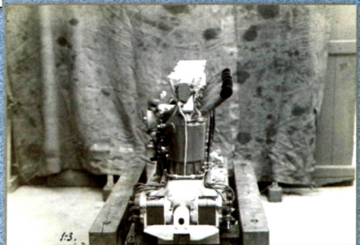
Рис. 3. 150-сильный двигатель конструкции Луцкого. Вид со стороны магнето (1914). Фотография из архива РАН
