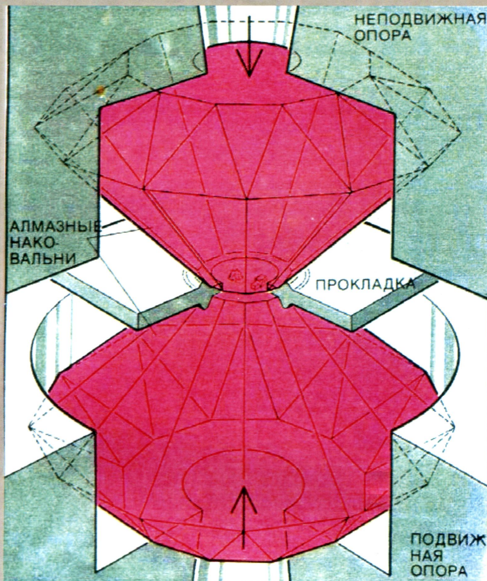
Рис. 4. Устройство алмазных наковален
