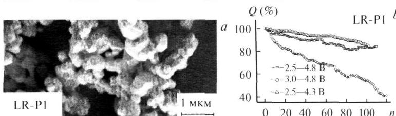
(a) Микроснимок (СЭМ) и (b) результаты циклирования лучшего образца в разных интервалах напряжения.
