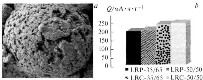
(a) Полученное методом СЭМ изображение для образца LRC-50/50 и (b) диаграмма разрядной емкости для первого цикла циклирования в диапазоне 2.5–4.8 В.
