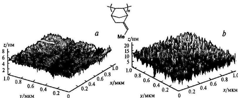
Поверхность полимерной пленки до (а) и после (b) модифицирования.
