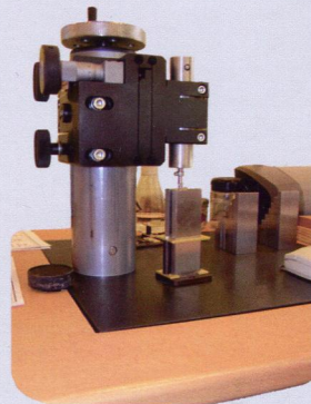
Установка для поверки концевых мер длины УКМ-100
