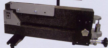
Экзаменатор эталонный I разряда М-055
