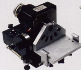
Прибор для поверки квадрантов ППК
