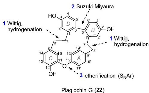
Plagiochin G (22)
